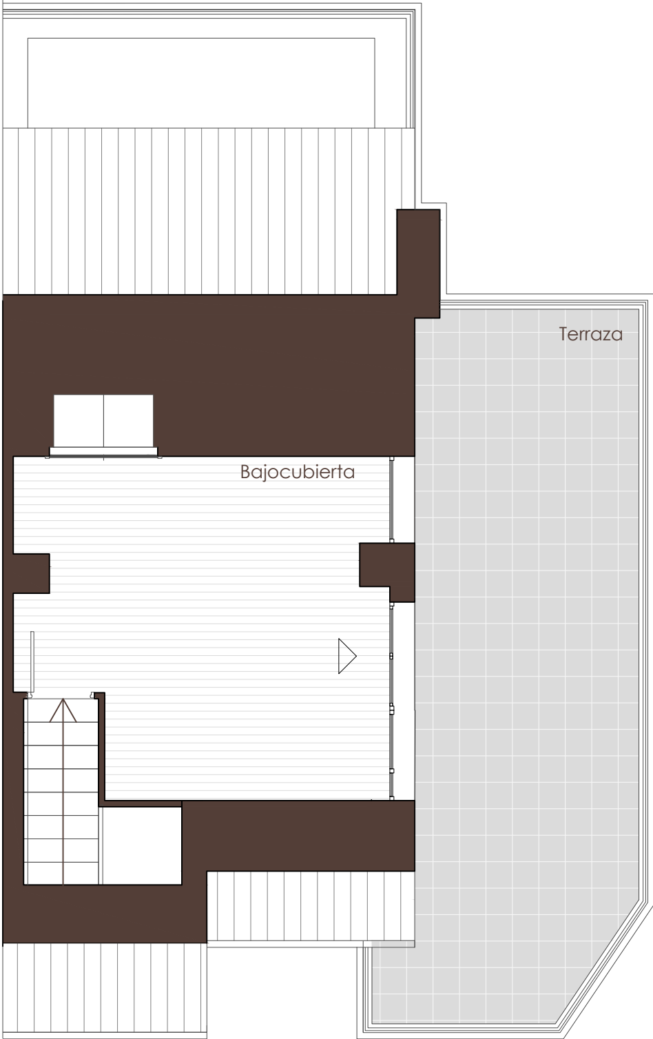
PLANTA BAJOCUBIERTA
