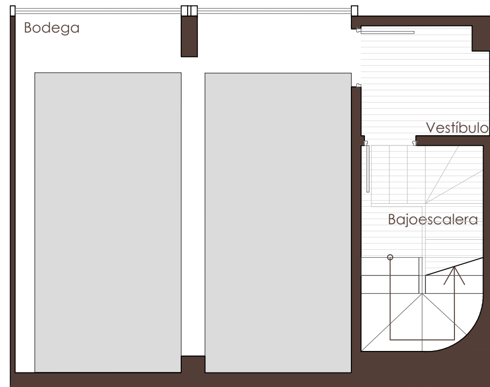
PLANTA SÓTANO
